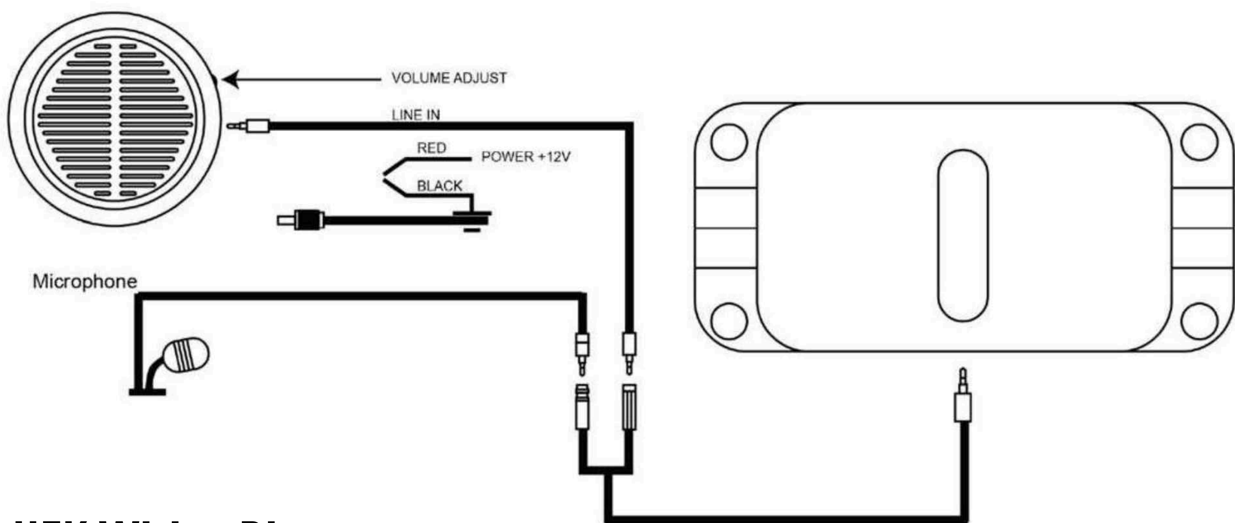
HFK Wiring Diagram
